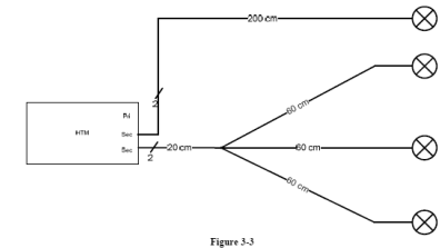
Parallelschaltung
